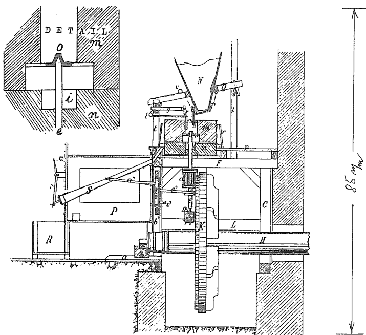
Schema mlýnského složení (3)
